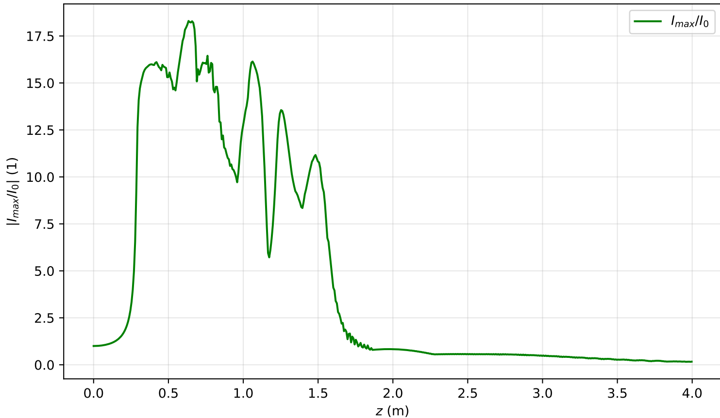
I_{\max}(r=0, z)/I_0 , Pin=9.8Pcr
